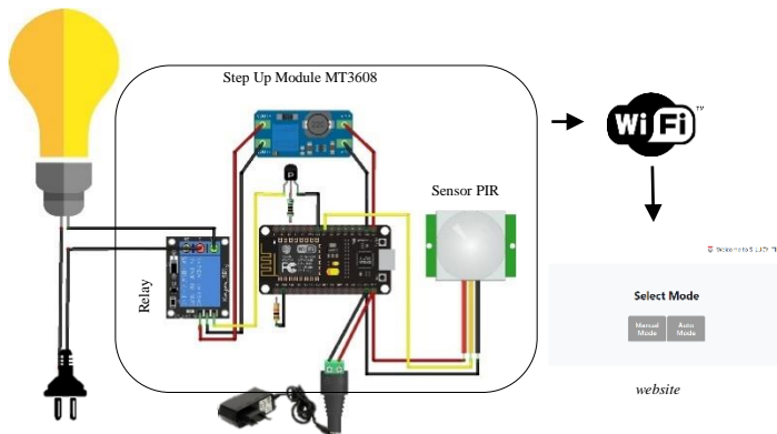
Gambar 1. Model Perancangan S-LUCY Smart Switch
